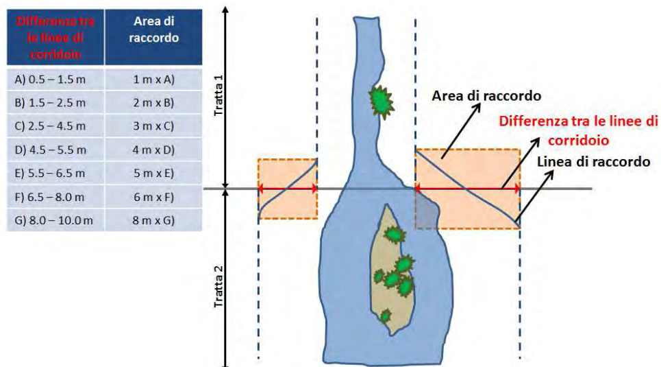
Figura 12: area e linea di raccordo
